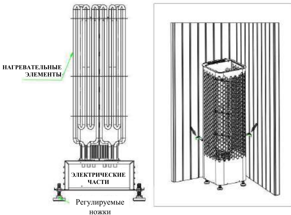
Рисунок 8. Установка каменки
