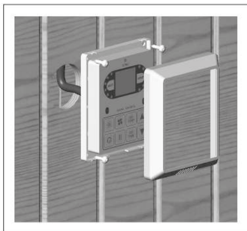
Схема 2. Установка панели управления
